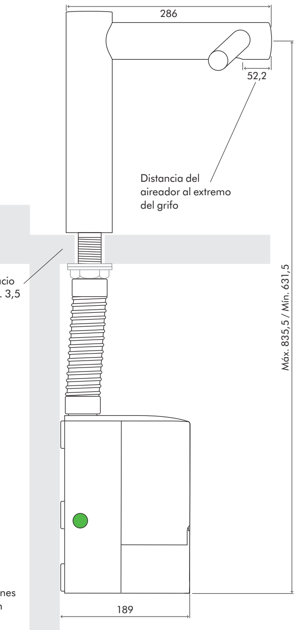
ALZADO LATERAL
