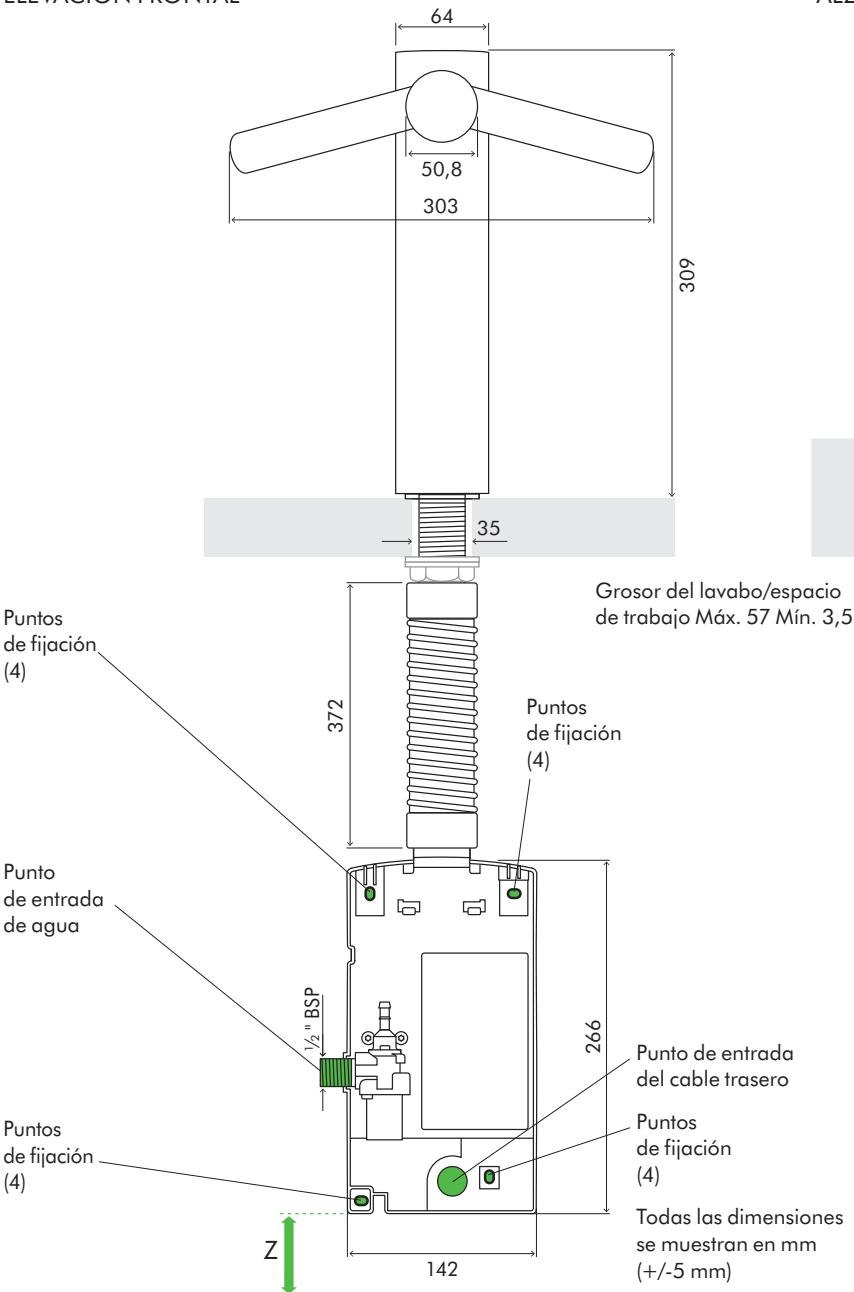
ELEVACIÓN FRONTAL
