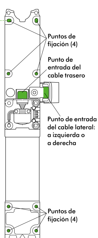
Placa trasera
